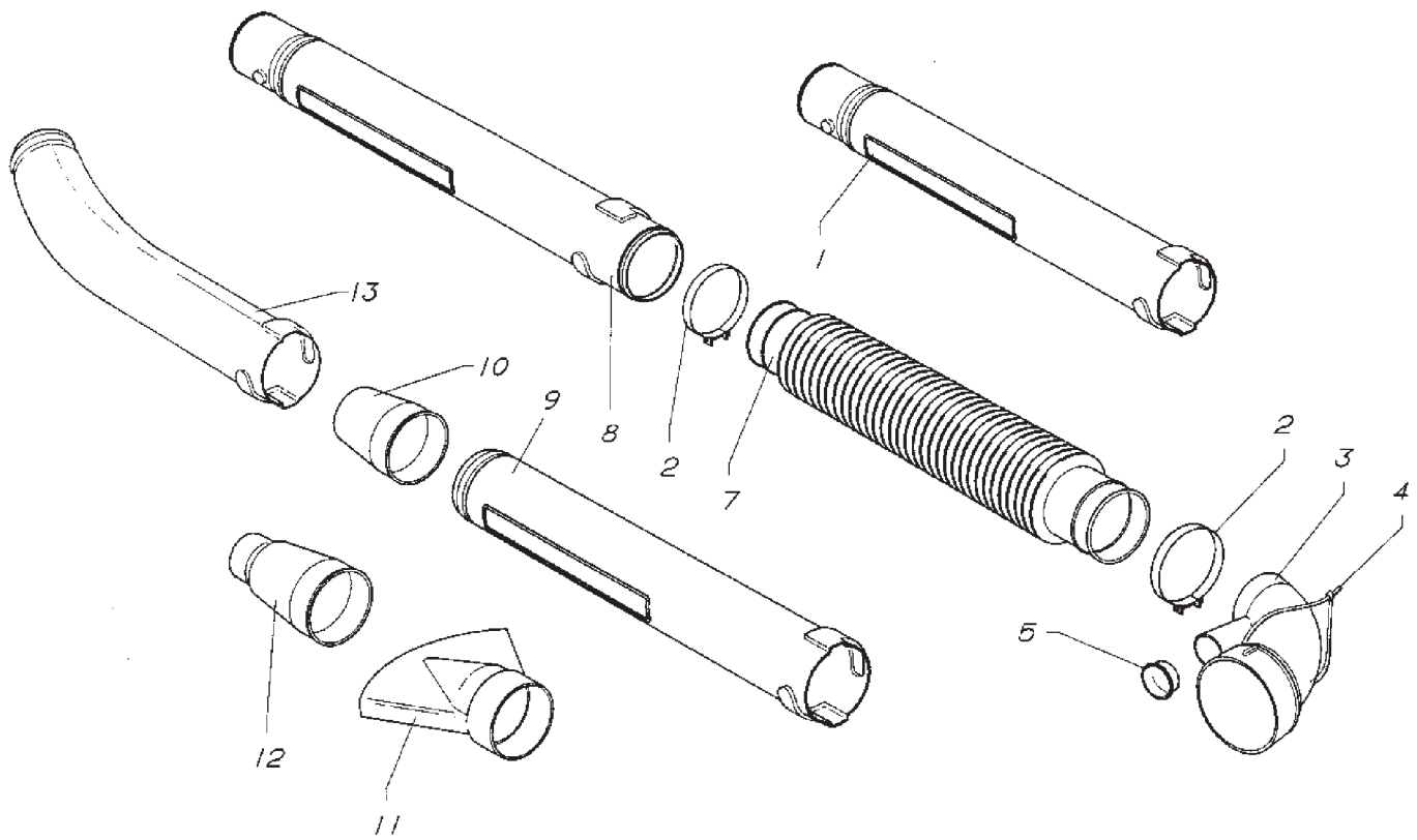
FIG.02 TUBO A
