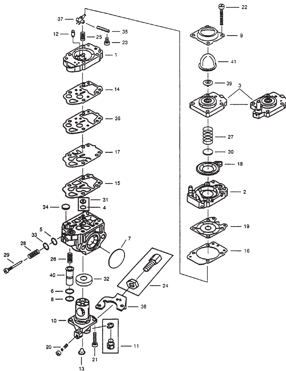
FIG.01 CARBURADOR
