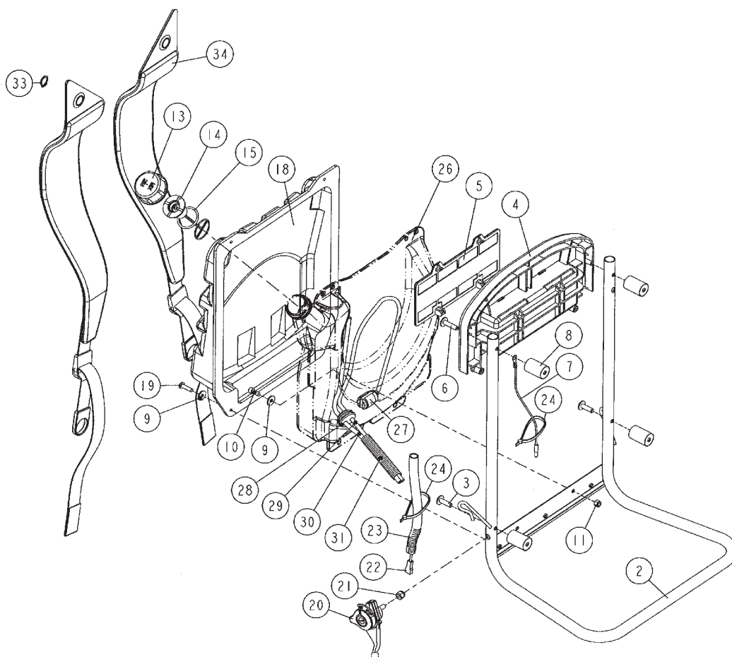
FIG.05 SUPORTE COSTAL
