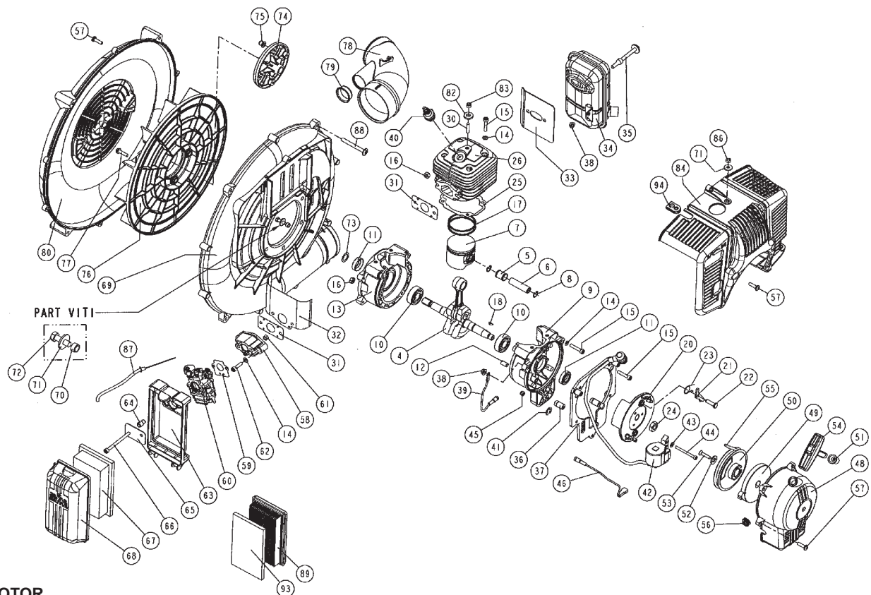
FIG.04 MOTOR
