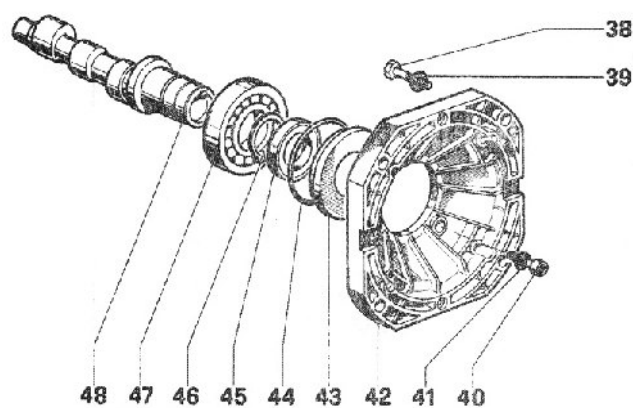
FIG.01 REDUTOR A
