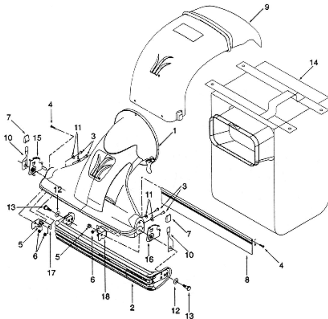
FIG.03 ASPIRACAO
