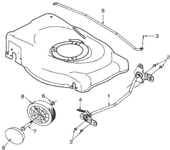
FIG.01 CORTADOR
