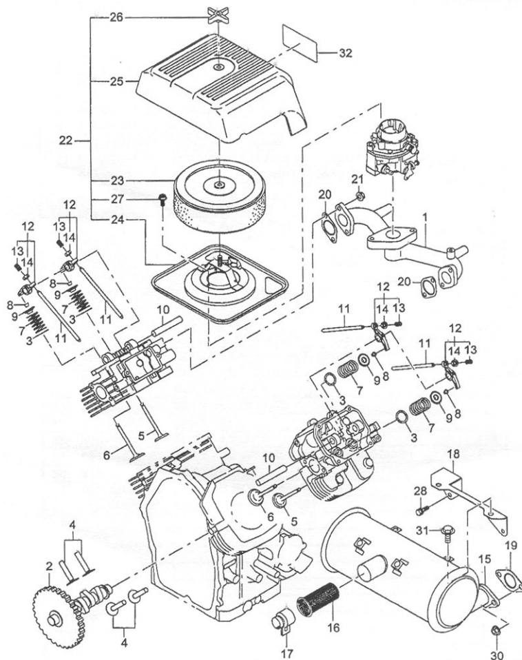
FIG.08 ADMISSÃO E EXAUSTÃO
