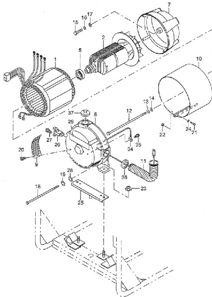
FIG.01 GRUPO GERADOR
