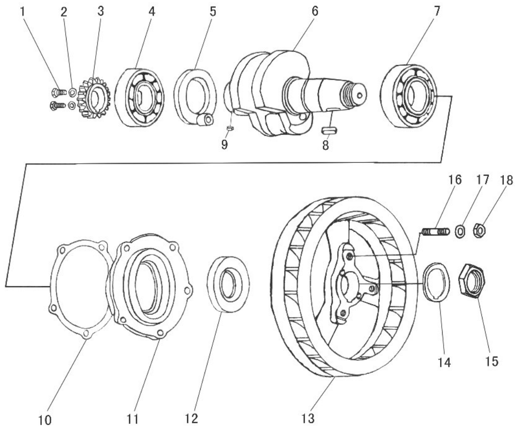
FIG.05 VOLANTE E VIRABREQUIM
