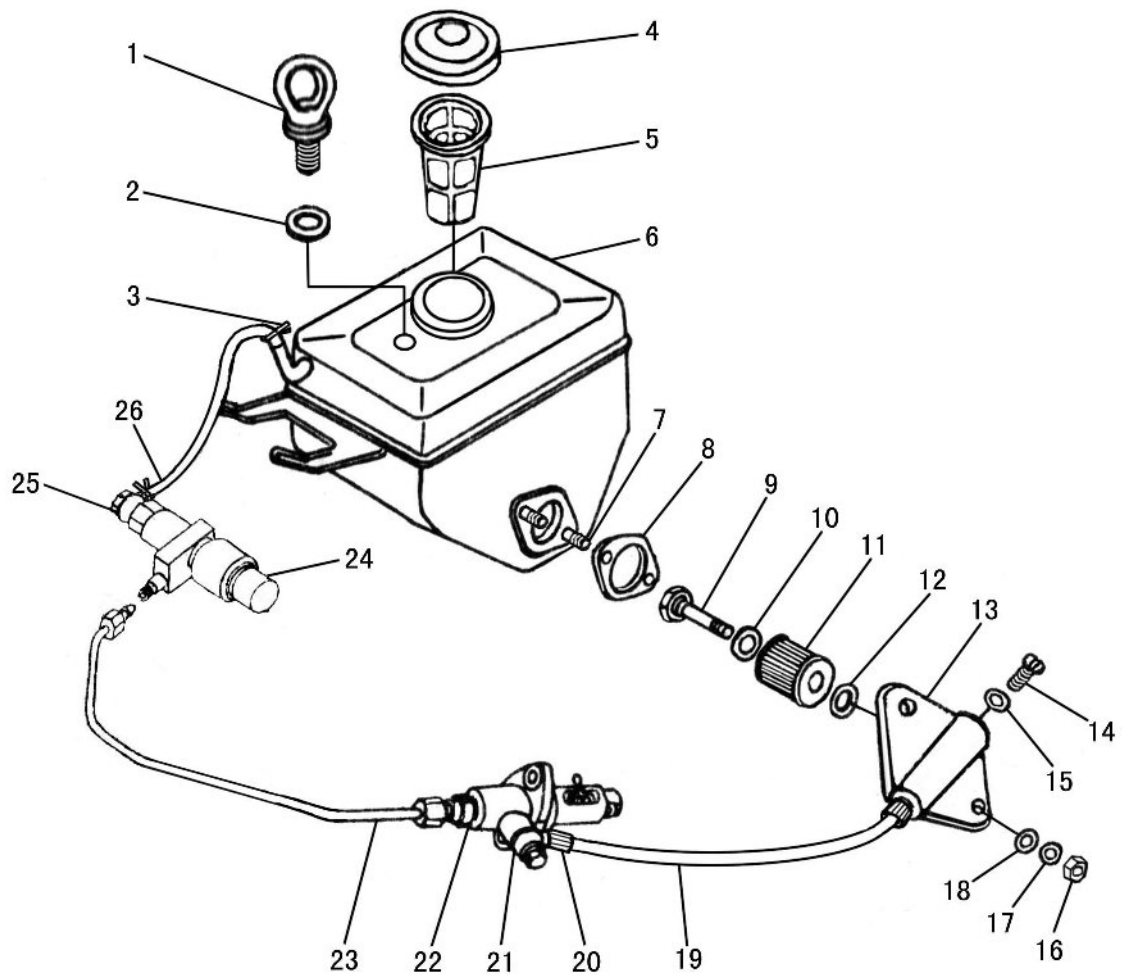
FIG.10 SISTEMA DE INJEÇÃO
