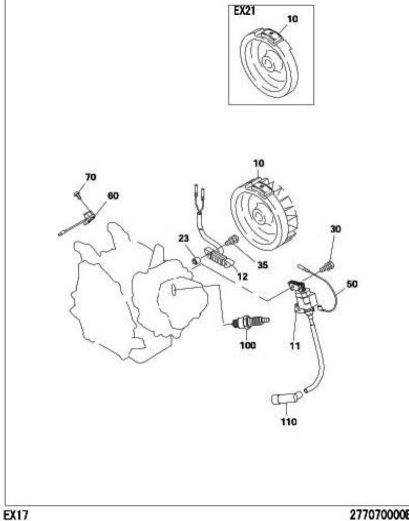
FIG.700 SISTEMA ELETRICO
