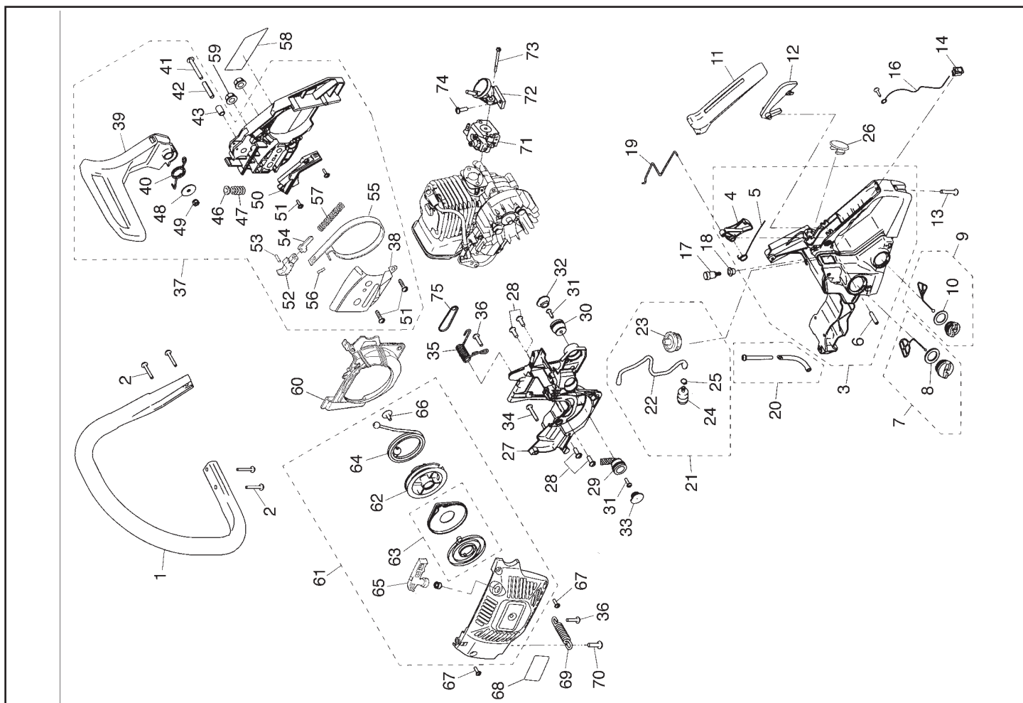
FIG.02 CARÇAÇA
