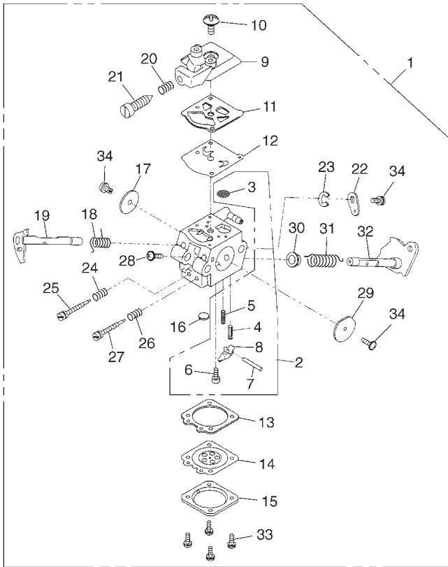
FIG.03 CARBURADOR
