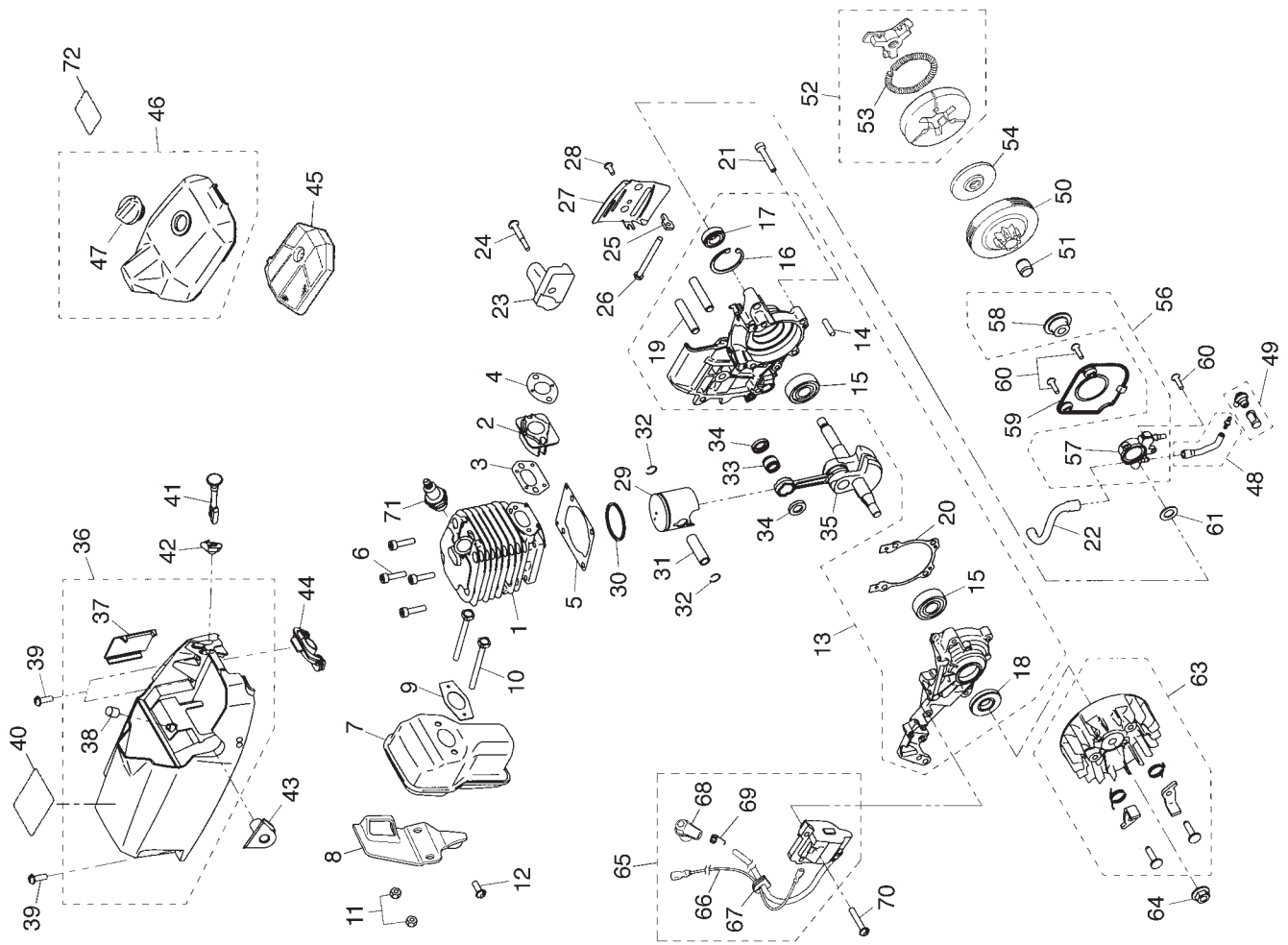
FIG.01 CONJUNTO TRASMISSÃO
